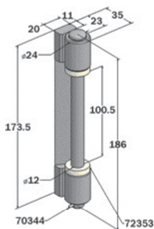
▲ Bolt-on hinge bracket
